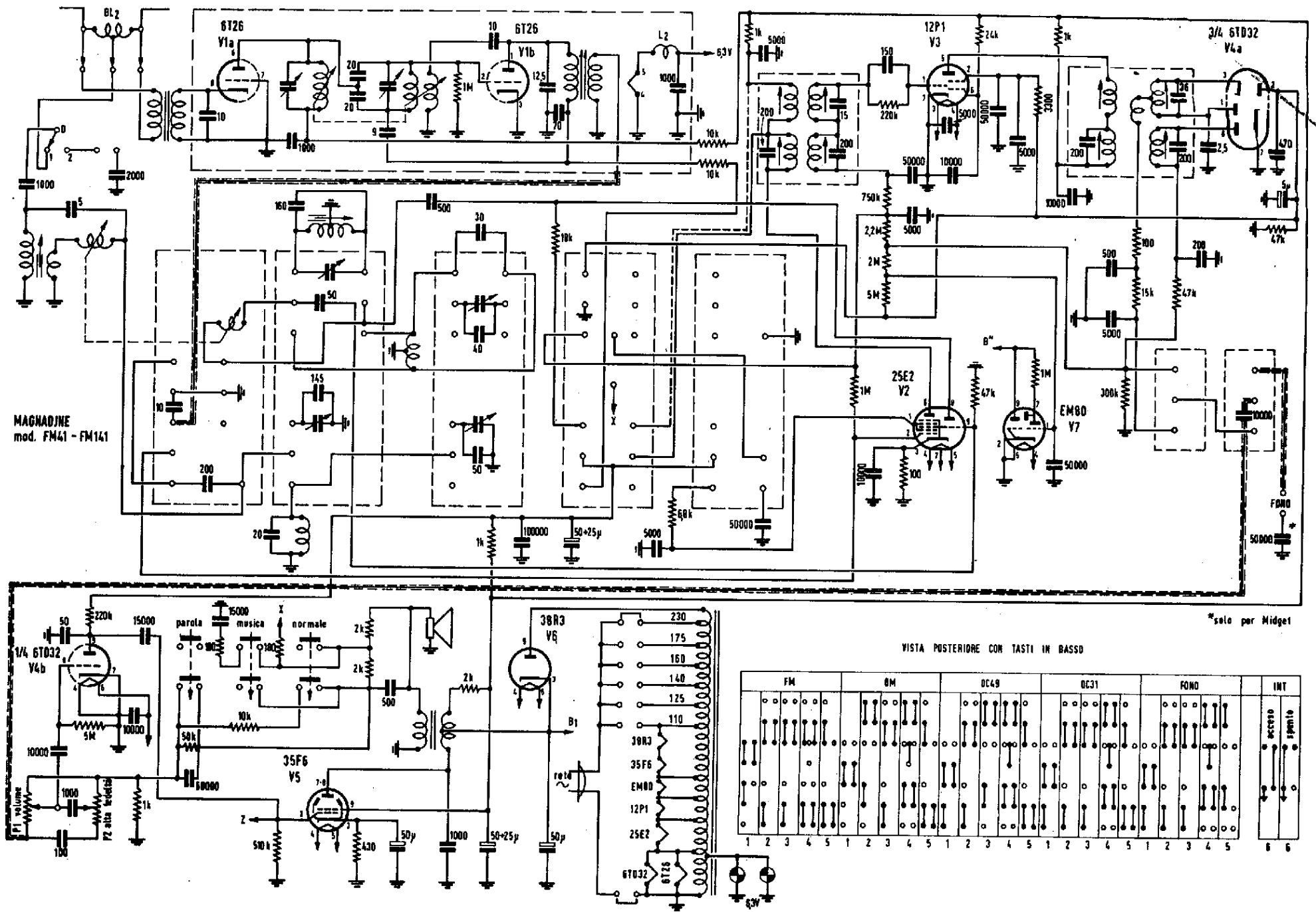
SCHEMA ELETTRICO DEL RADIORICEVITORE AM-FM, MAGNADYNE, MOD. FM41 . FM141
